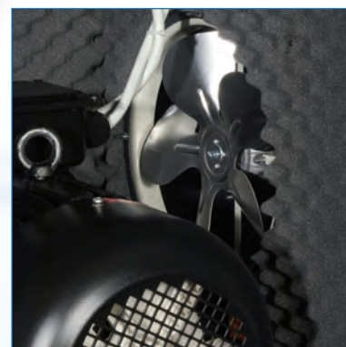
Koeling met extra elektrische ventilator (op 7,5 en 10 PK)
